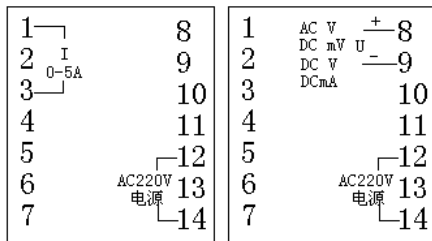
交流电流表 交直流电压表，直流75mV
